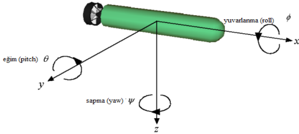
Şekil 3.1. OSA koordinat sistemi ve 6-DOF
