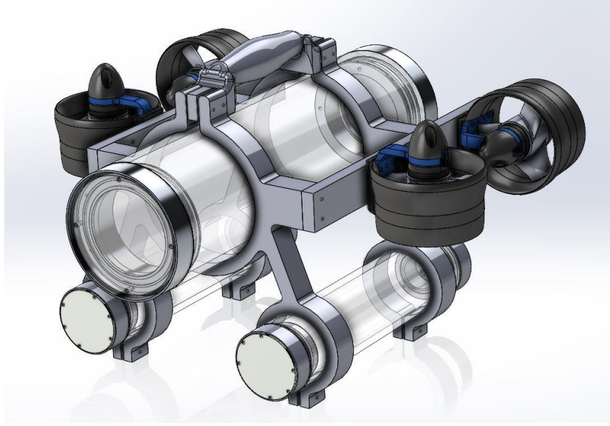
Şekil A. 1. RedFin gvde yapısı genel grnm
